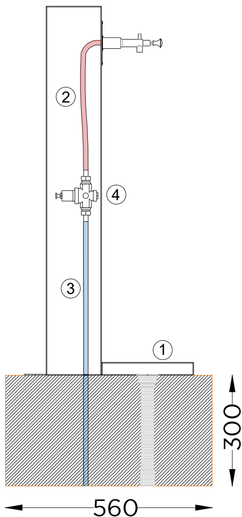
ALÇADO LAT. ESQUEMA DE FIXAÇÃO SIDE VIEW INSTALLATION PLAN
