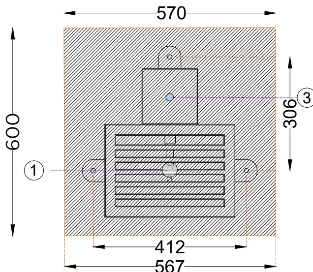
PLANTA . ESQUEMA DE FIXAÇÃO PLAN . INSTALLATION PLAN
