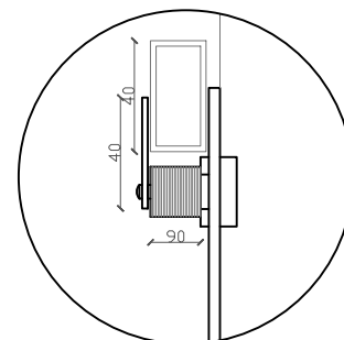
PORMENOR A (Esc. 5/1) Esquema de abertura na parte superior, através da chave da papeleira.
