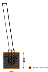
ESQUEMA DE FIXAÇÃO CHUMBADOURO FIXATION SCHEME ANCHOR BOLT
