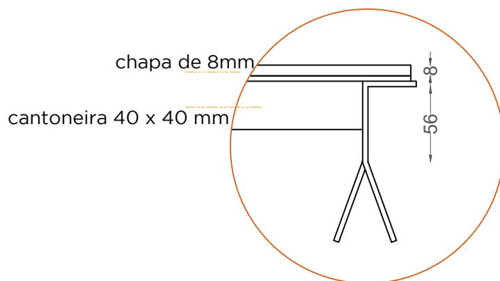
ALÇADO FRONTAL FRONT VIEW
