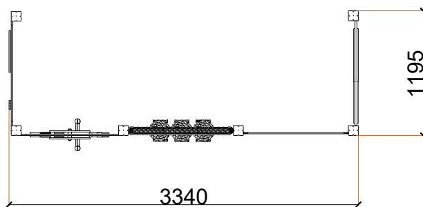
PLANTA PLAN
