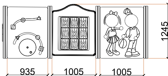
ALÇADO LATERAL SIDE VIEW
