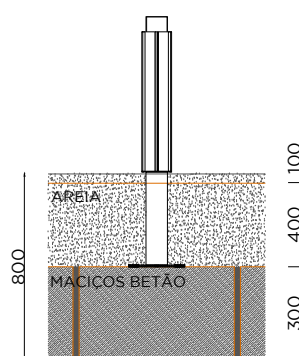
MACIÇO BETÃO + PISO AREIA
