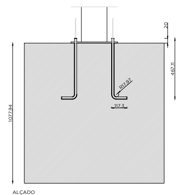
ALÇADO
