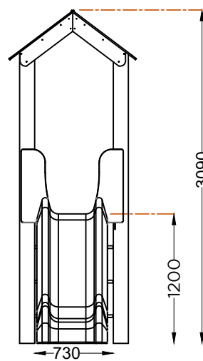
ALÇADO FRONTAL FRONT VIEW
