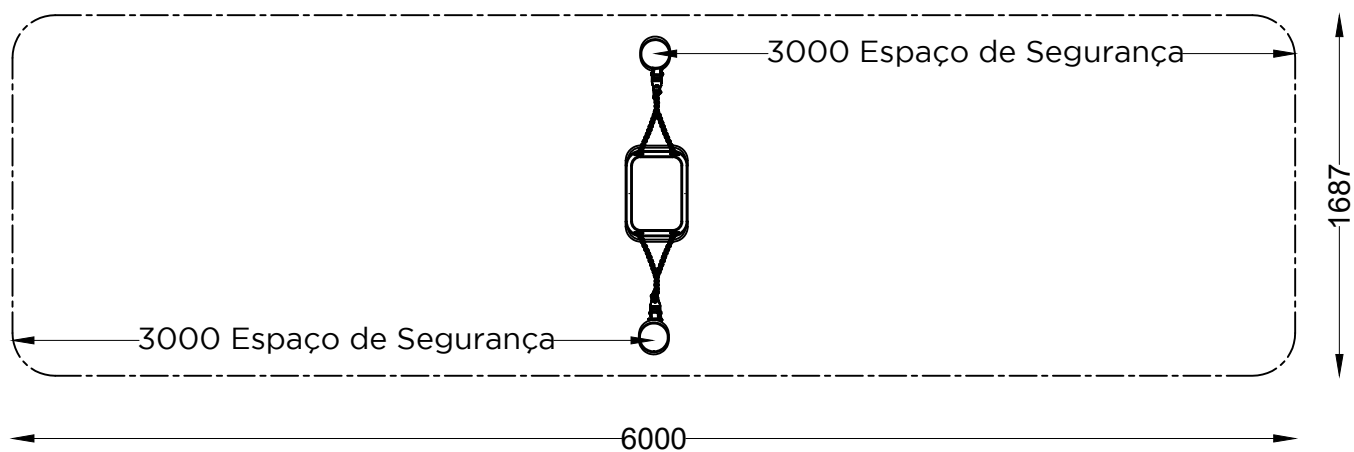
PLANTA - ESPAÇO DE SEGURANÇA NECESSÁRIO PLAN - SAFETY SPACE REQUIRED
