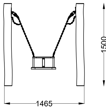
ALÇADO FRONTAL FRONT VIEW
