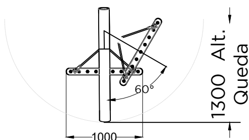
ALÇADO LATERAL SIDE VIEW
