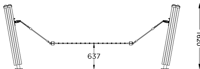
ALÇADO FRONTAL FRONT VIEW
