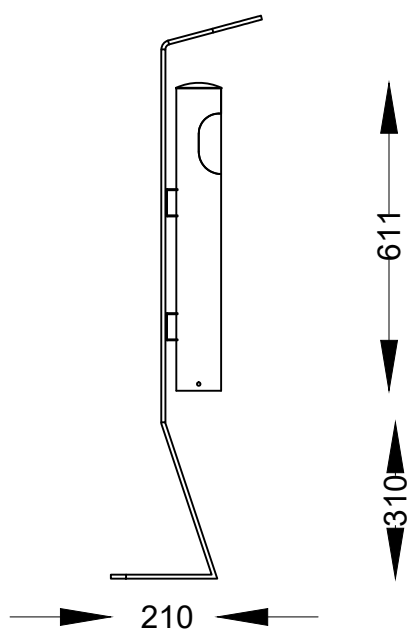
ALÇADO LATERAL SIDE VIEW
