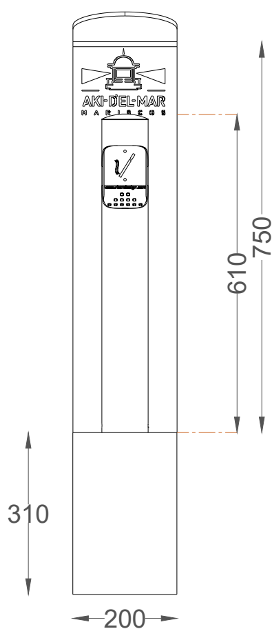
ALÇADO FRONTAL FRONT VIEW
