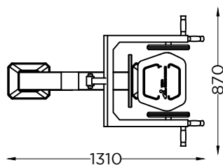
PLANTA PLAN
