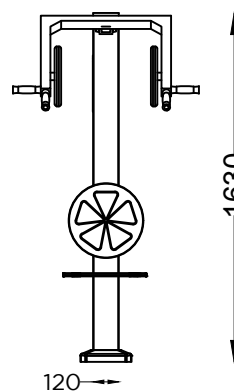
ALÇADO FRONTAL FRONT VIEW
