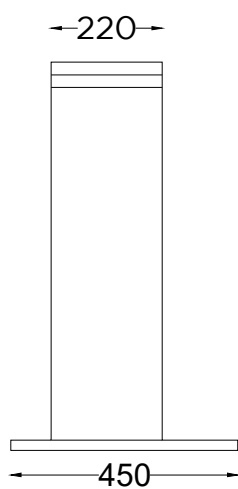
ALÇADO LATERAL SIDE VIEW
