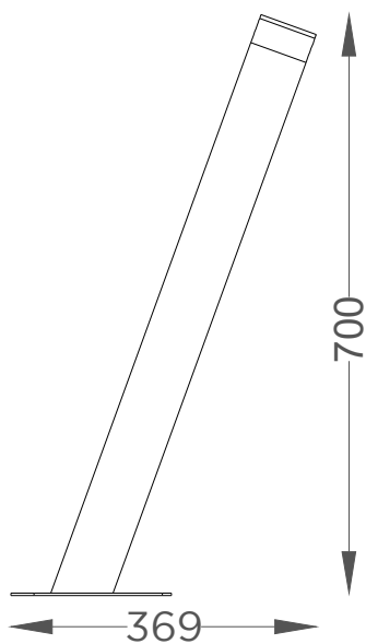
ALÇADO LATERAL SIDE VIEW
