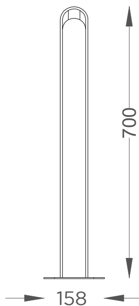
ALÇADO FRONTAL FRONT VIEW
