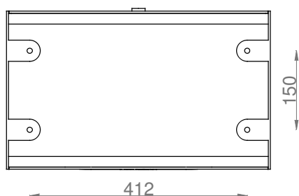
PLANTA INFERIOR
