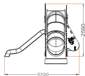
ALÇADO FRONTAL FRONT VIEW
