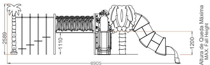
ALÇADO LATERAL SIDE VIEW
