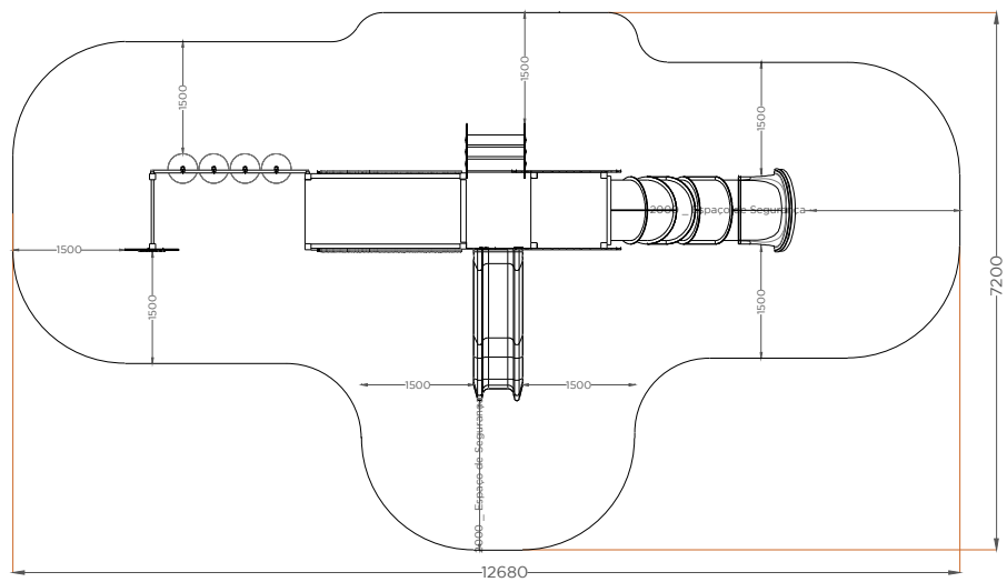
PLANTA - ESPAÇO DE SEGURANÇA NECESSÁRIO PLAN - SAFETY SPACE REQUIRED
