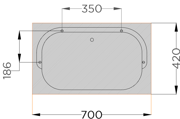
PLANTA . ESQUEMA DE FIXAÇÃO PLAN . INSTALLATION PLAN
