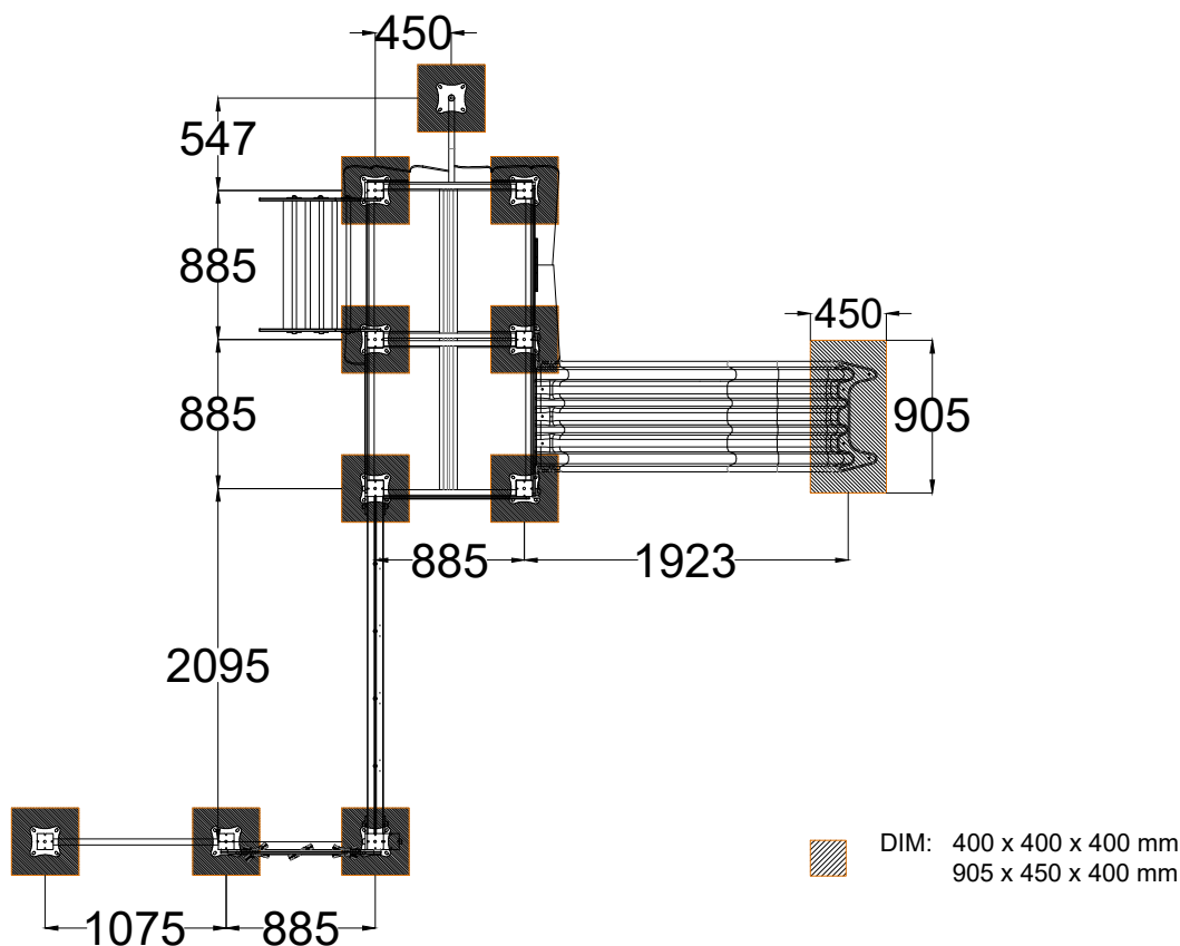
PLANTA . ESQUEMA DE FIXAÇÃO PLAN . INSTALLATION PLAN
