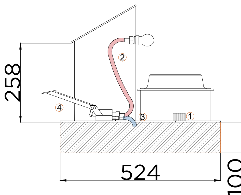
ALÇADO
