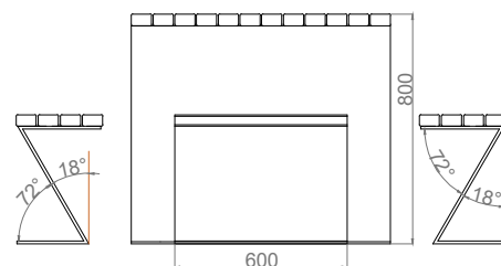
ALÇADO LATERAL
