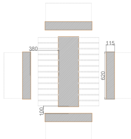
PLANTA - ESQUEMA DE MACIÇOS
