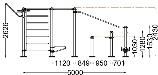
ALÇADO FRONTAL FRONT VIEW
