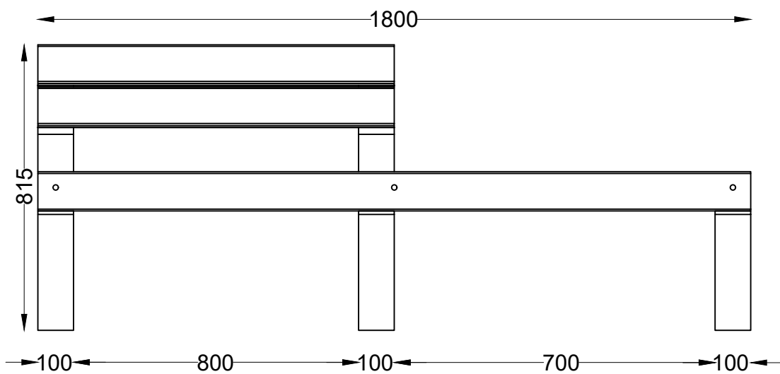
ALÇADO FRONTAL FRONT VIEW
