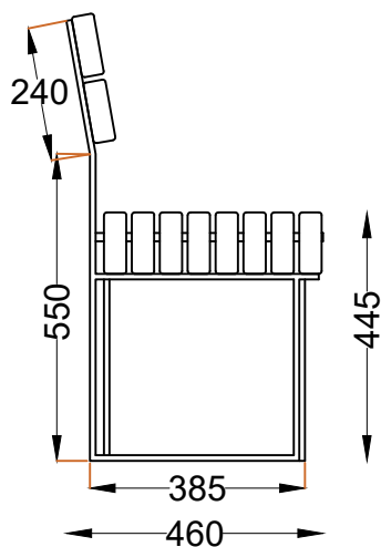
ALÇADO LATERAL SIDE VIEW
