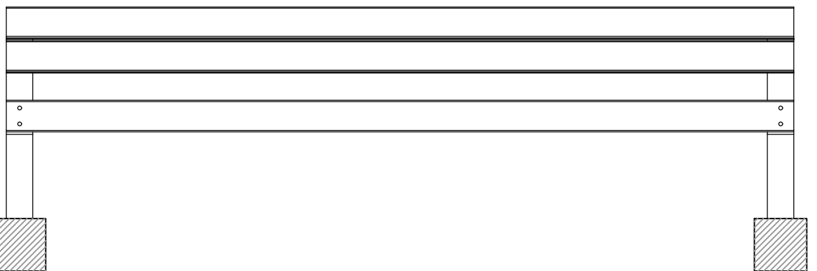
ALÇADO FRONTAL
