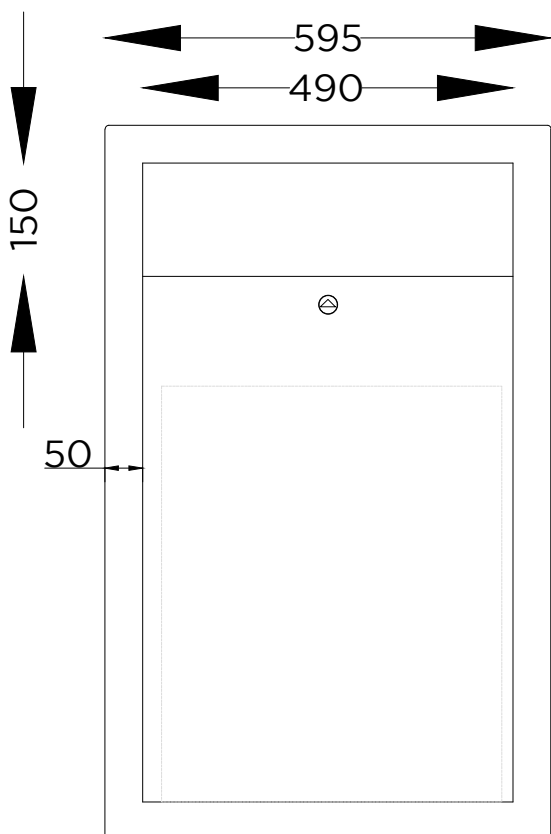
ALÇADO FRONTAL FRONT VIEW
