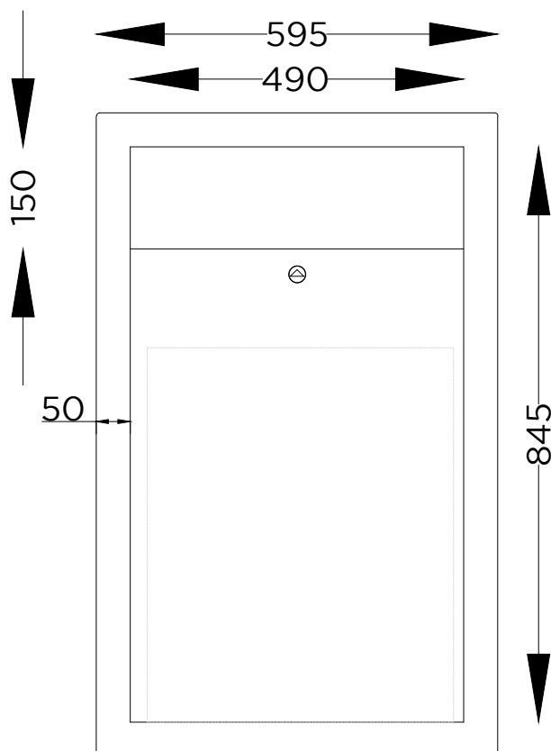
ALÇADO FRONTAL FRONT VIEW
