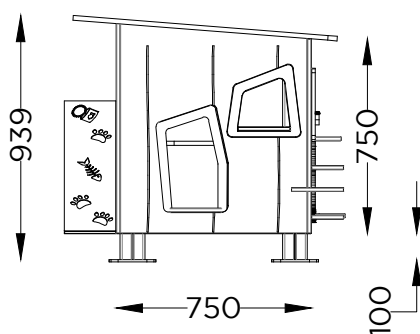
ALÇADO LATERAL SIDE VIEW
