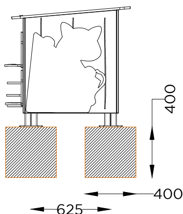
ALÇADO FRONTAL. ESQUEMA DE FIXAÇÃO FRONT VIEW . INSTALLATION PLAN
