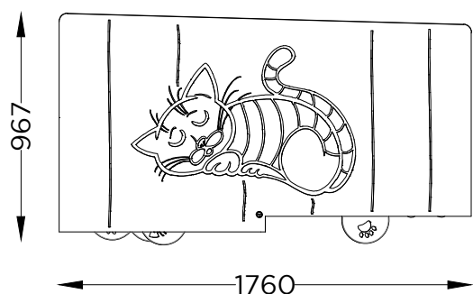
PLANTA PLAN
