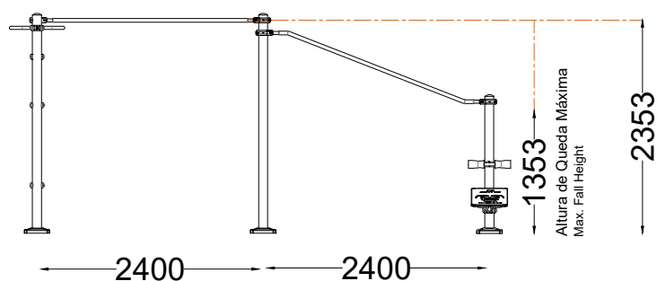
ALÇADO LATERAL SIDE VIEW
