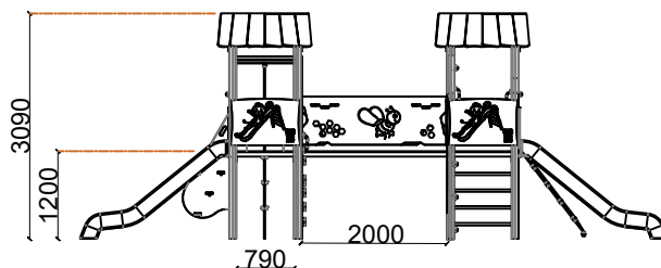
ALÇADO LATERAL SIDE VIEW
