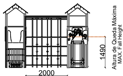
ALÇADO FRONTAL FRONT VIEW
