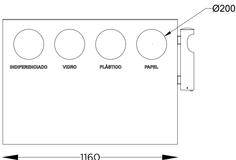
ALÇADO FRONTAL FRONT VIEW
