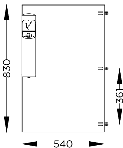
ALÇADO LATERAL SIDE VIEW
