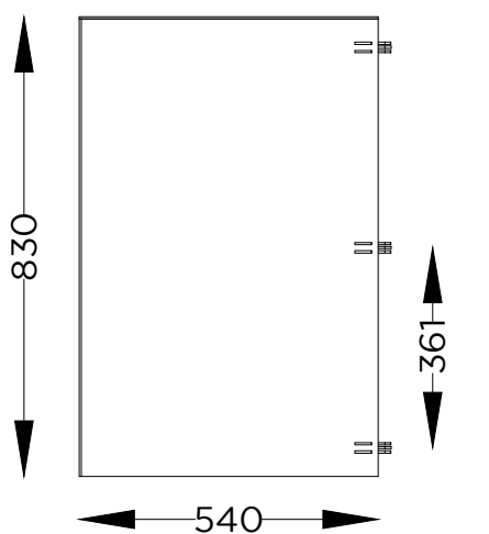
ALÇADO LATERAL SIDE VIEW
