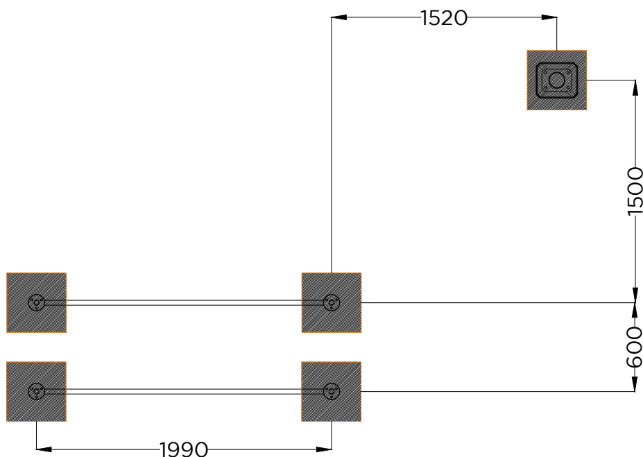
PLANTA . ESQUEMA DE FIXAÇÃO PLAN . INSTALLATION PLAN
