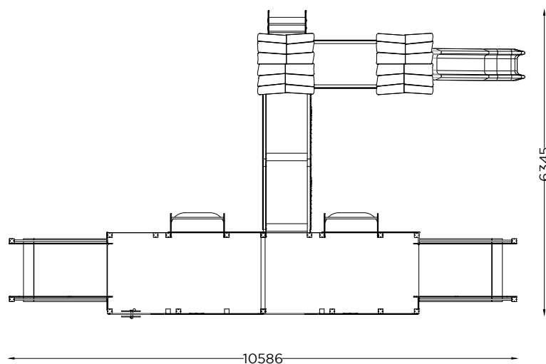
PLANTA PLAN
