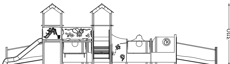
ALÇADO LATERAL SIDE VIEW
