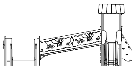
ALÇADO FRONTAL FRONT VIEW
