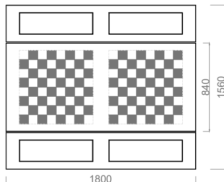
PLANTA
