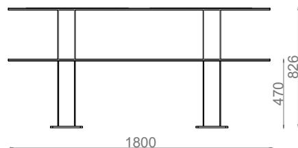
ALÇADO FRONTAL
