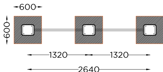
PLANTA . ESQUEMA DE FIXAÇÃO PLAN . INSTALLATION PLAN
