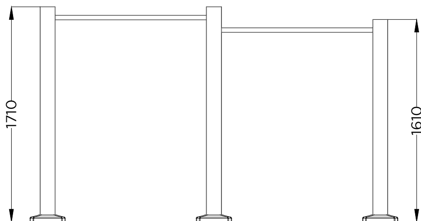
ALÇADO FRONTAL FRONT VIEW
