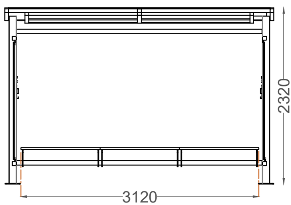
ALÇADO FRONTAL FRONT VIEW
