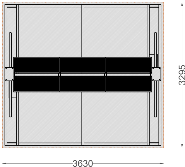
PLANTA . ESQUEMA DE FIXAÇÃO EM BASE DE BETÃO PLAN . INSTALLATION PLAN IN CONCRETE BASE
