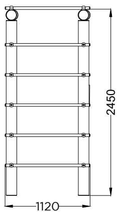
ALÇADO FRONTAL FRONT VIEW
