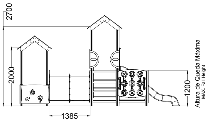
ALÇADO LATERAL SIDE VIEW
