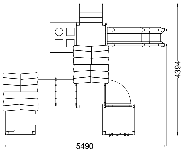
PLANTA PLAN
