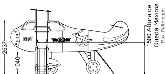
ALÇADO LATERAL SIDE VIEW
