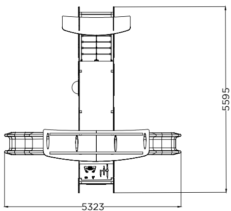
PLANTA PLAN
