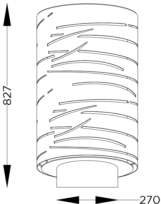
ALÇADO LATERAL SIDE VIEW
