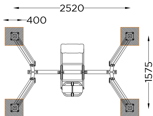
PLANTA . ESQUEMA DE MACIÇOS
