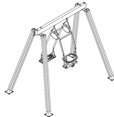
VISTA ISOMÉTRICA
