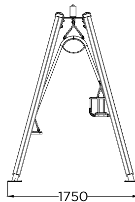
ALÇADO LATERAL
