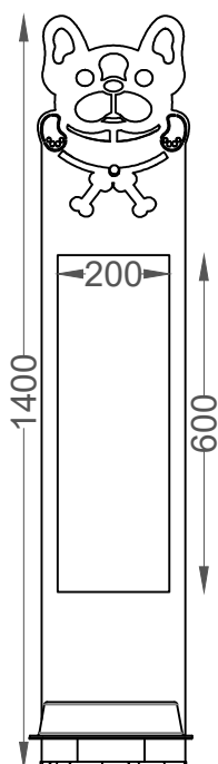
ALÇADO FRONTAL FRONT VIEW
