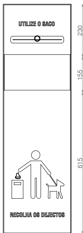
ALÇADO FRONTAL
