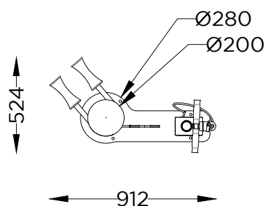
PLANTA PLAN
