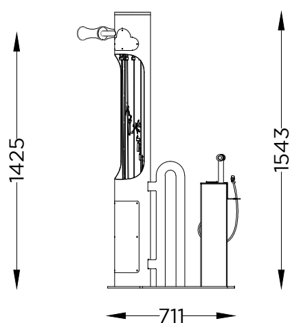
ALÇADO FRONTAL FRONT VIEW
