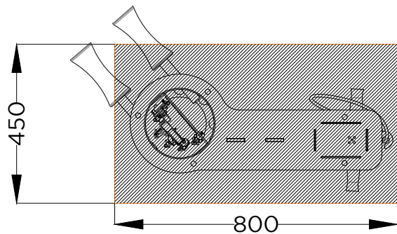
PLANTA . ESQUEMA DE FIXAÇÃO PLAN . INSTALLATION PLAN
