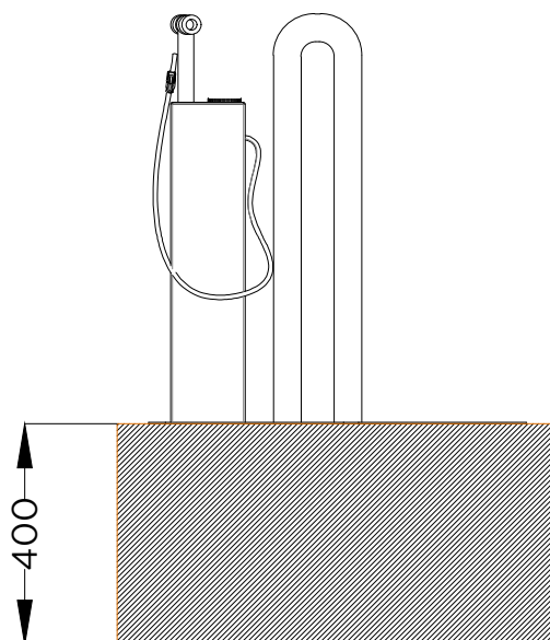
PLANTA . ESQUEMA DE FIXAÇÃO PLAN . INSTALLATION PLAN
