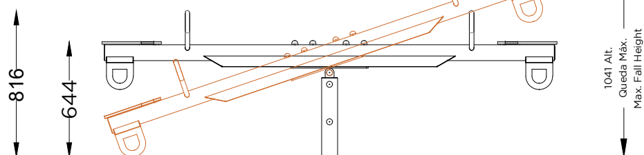
ALÇADO FRONTAL FRONT VIEW
