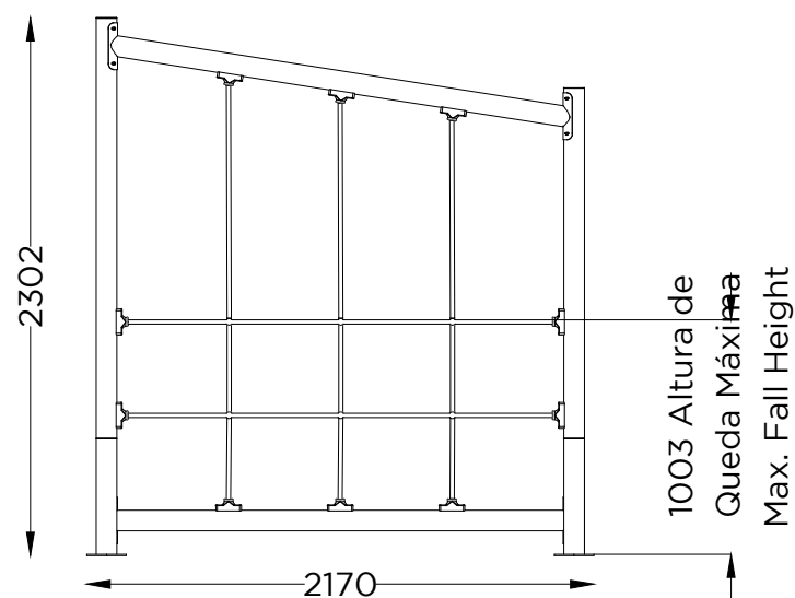
ALÇADO FRONTAL FRONT VIEW
