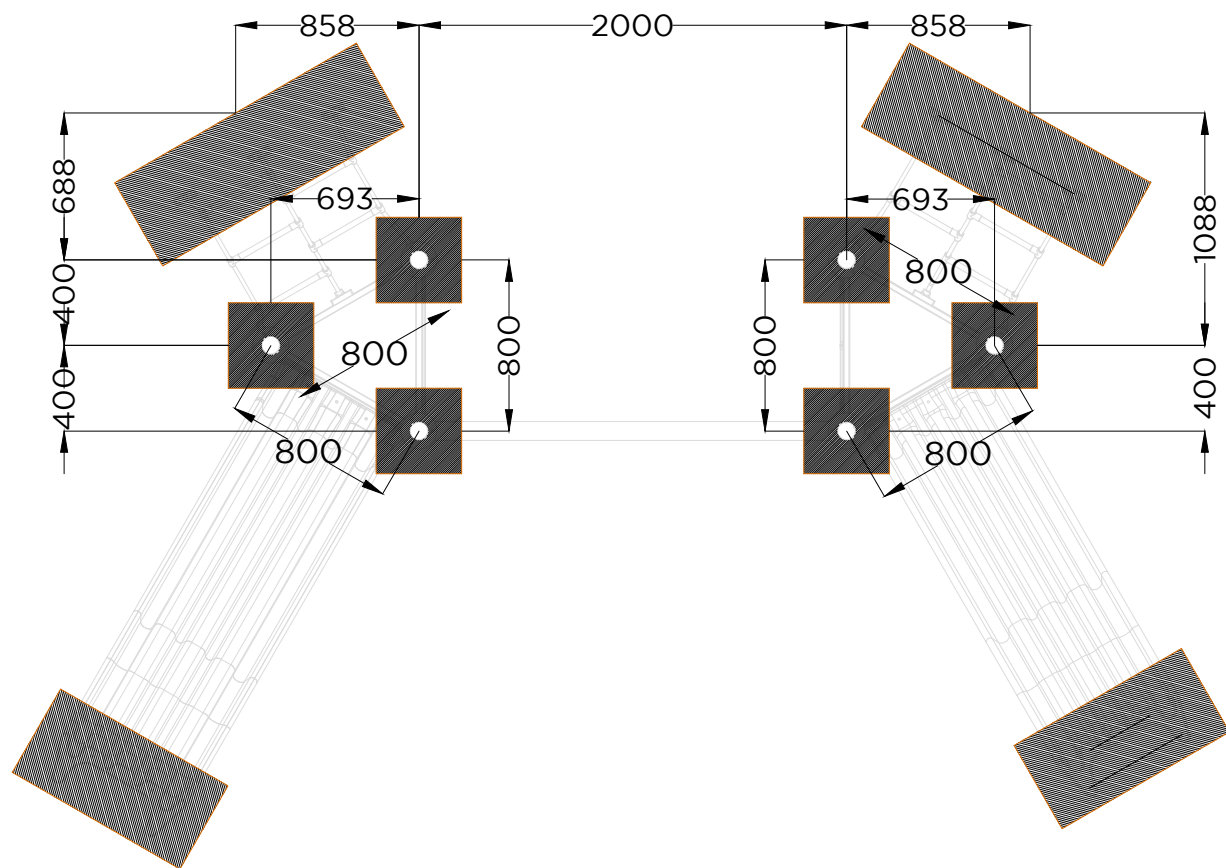
PLANTA . ESQUEMA DE FIXAÇÃO PLAN . INSTALLATION PLAN
