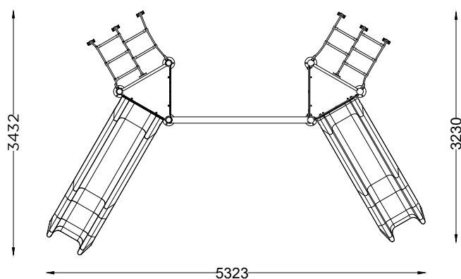
PLANTA PLAN
