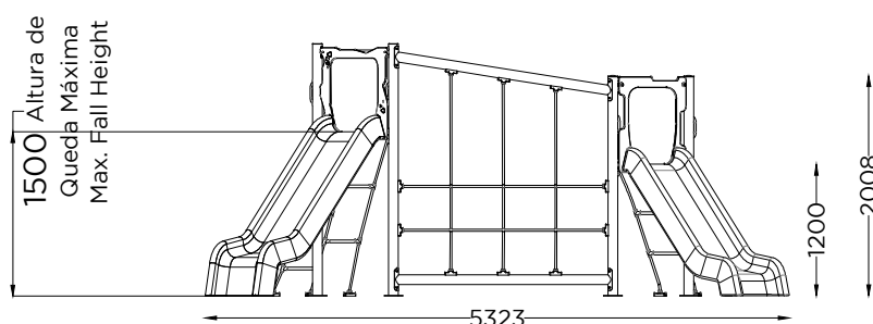
ALÇADO FRONTAL FRONT VIEW
