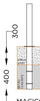
MACIÇO BETÃO + PISO AREIA P/ENTERRAMENTO CONCRETE BLOCK + SAND LAYER BY BURIAL
