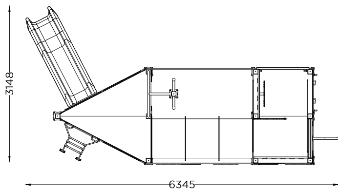
PLANTA PLAN
