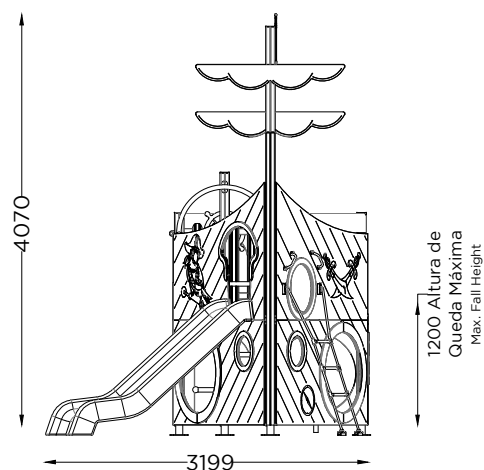
ALÇADO LATERAL SIDE VIEW
